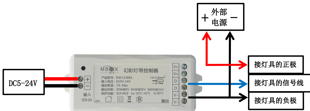
RW-LC240C 接“外部电源+” “外部电源-” “输出 D” “输出 V-”
