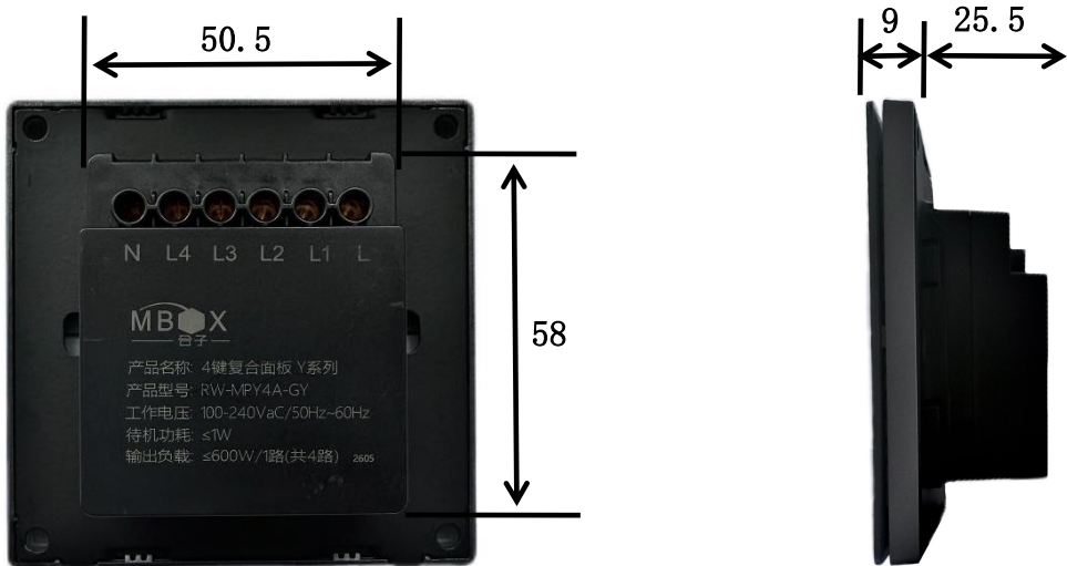
A*B*C=50.5*58*25.5 Unit:mm
